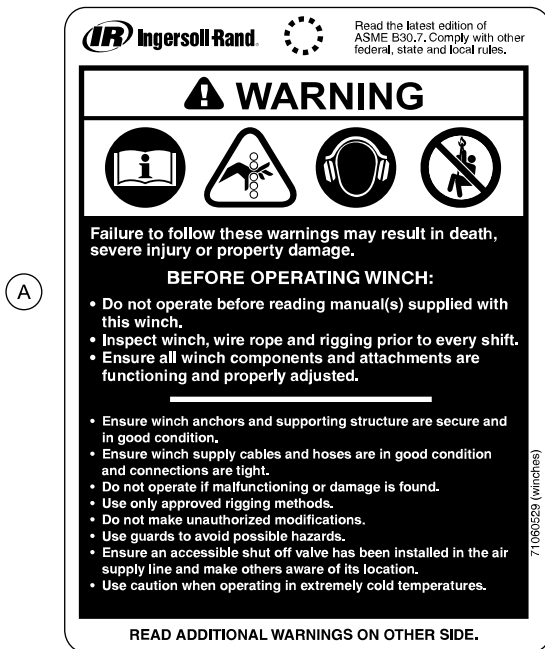
(Desenho 71060529)
