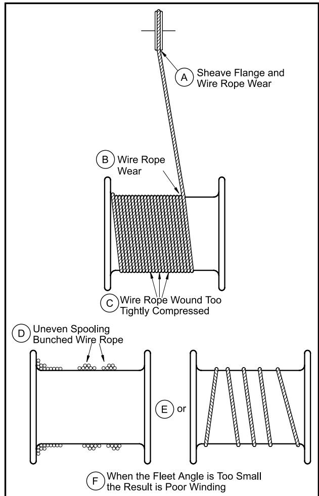
(Dwg. MHP2453)
